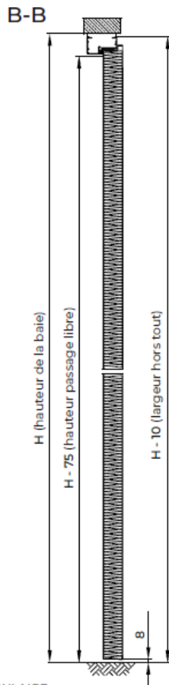
BÂTI TUBULAIRE
