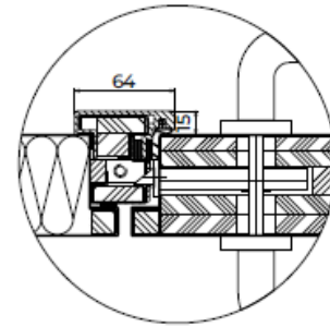
C - côté serrure plat de battent
