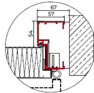
D - côté paumelles 3D
