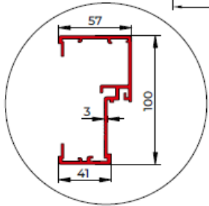
BÂTI TUBULAIRE
